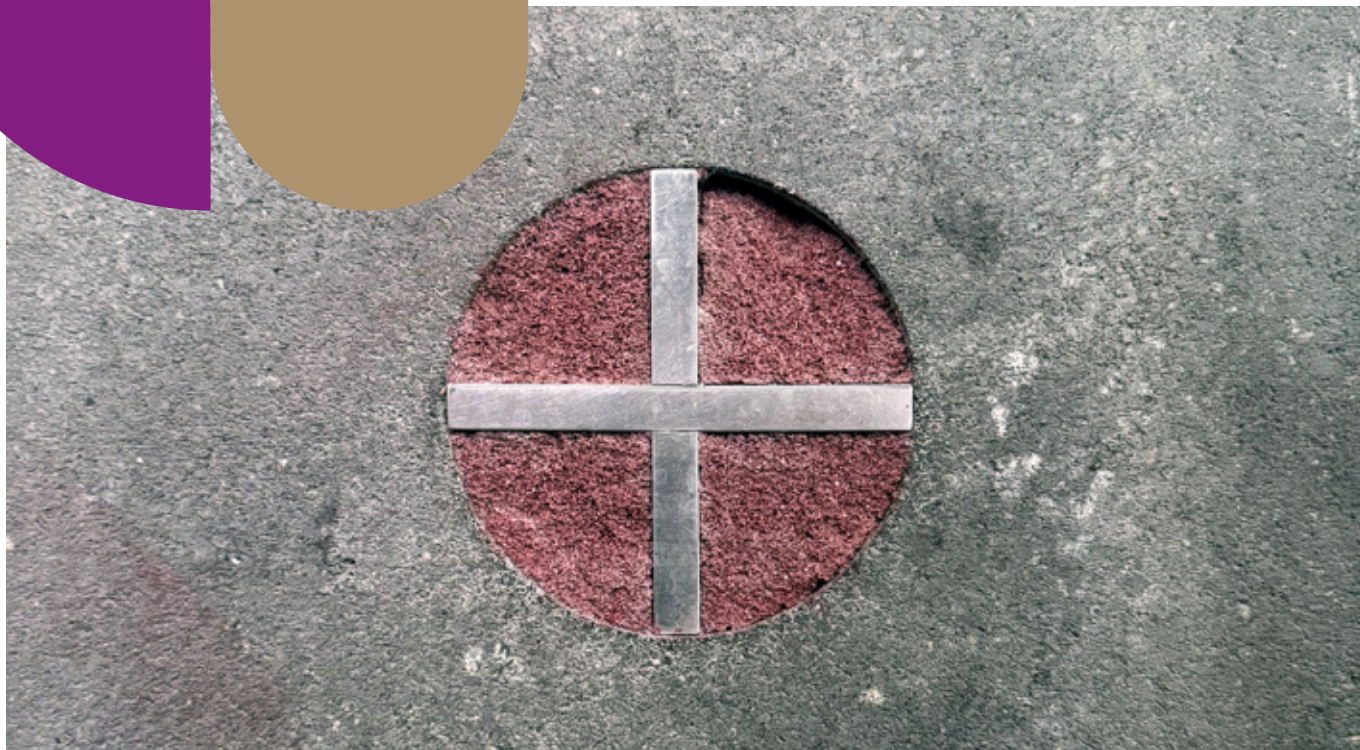
Stein vom Kreuzweg zum Muttergotteshäuschen: Edelstahlkreuz, nicht geschweißt, gesteckt. Füllung in Kreisform – Eisenoxidpigment mit Epoxidharz und gebrochenem Sand gemischt. Eingesetzt in eine mit Wasserstrahl geschnittene Gehwegplatte. Entwurf: Arno Günther Knott & Jan Philipp Koch.
